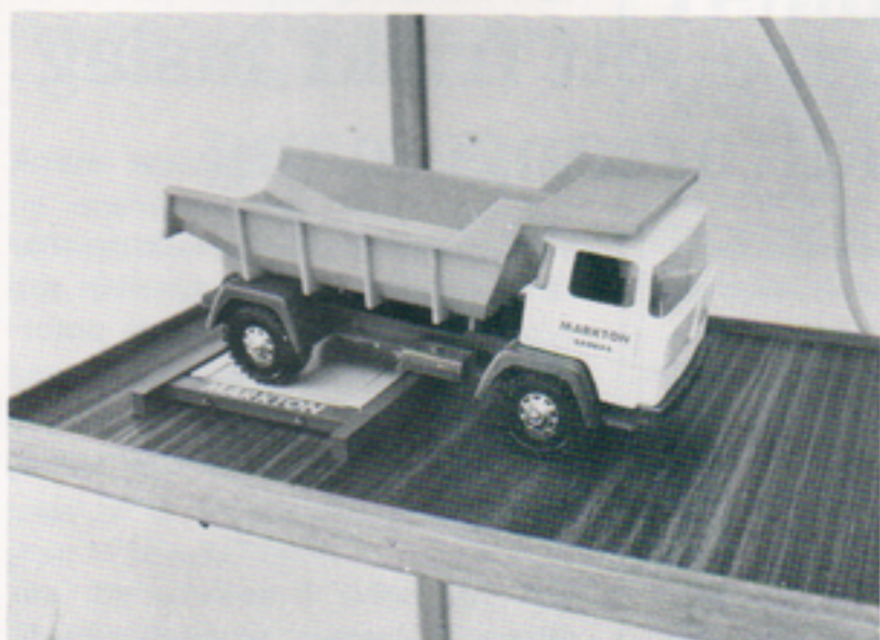
En modell av den dynamiska elektroniska fordonsvägen Markton, en axel- och boggietrycksvåg för max 30 ton.
