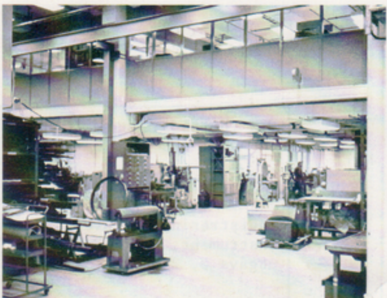
Den mekaniska verkstaden i nedre hallen är ännu inte helt klar vad inredningen beträffar. Den yttre delen — i förgrunden — är betydligt högre än den inre.
