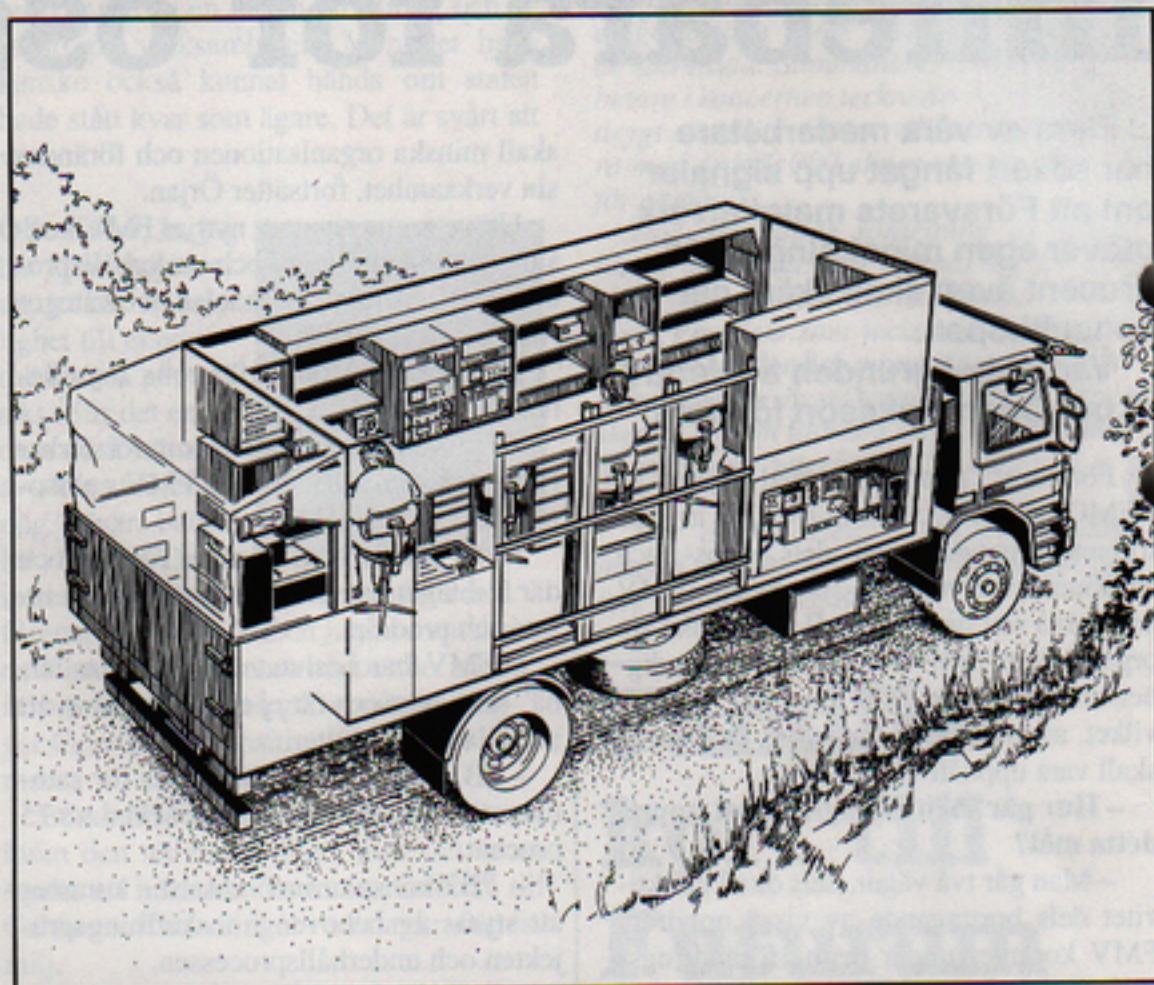
Telub Teleanläggningar har tagit fram prototypen till den här vagnen, som skall användas för reparation av telemateriel i krig och fred. Serieproduktionen startar nästa år på verkstäderna i Växjö.
