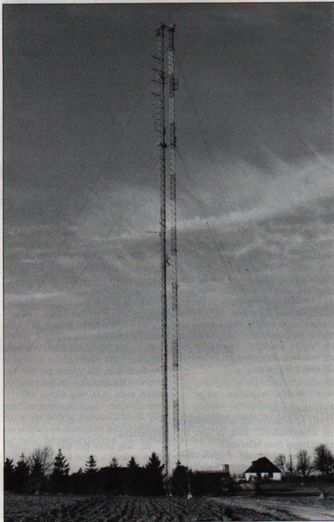
Den skånska slättens starka vindar sätter masterna på prov. Telub Teknik har här rest en ny SJ-mast, som tål orkanvindar upp till 48 meter per sekund. Den gamla, som nu har rivits, klarade inte de hårda kraven på stabilitet. Foto: Reinhold Carlsson
