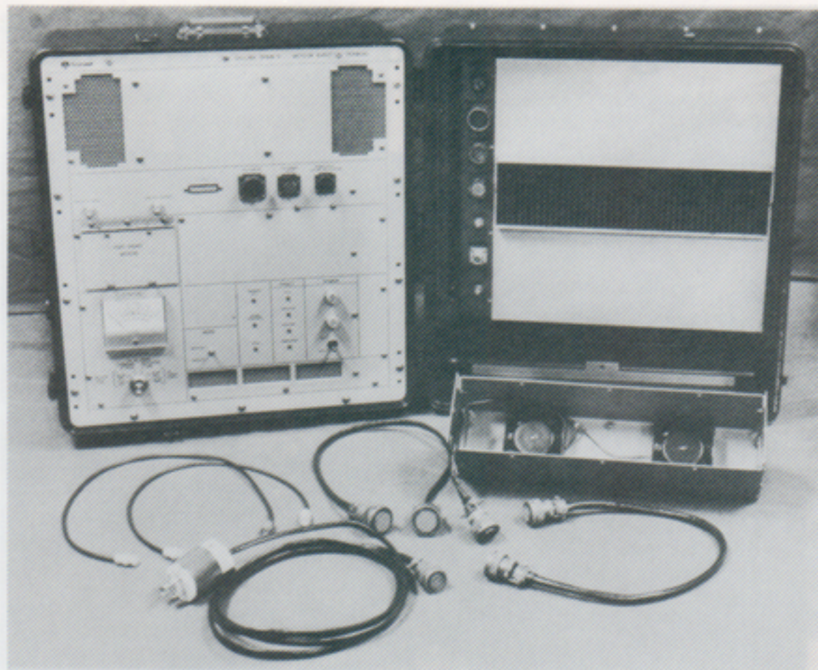
Utrustningen som skall användas i försöksverksamheten av FFV Elektronik och FOA i forskningen kring meteorspårkommunikation.
